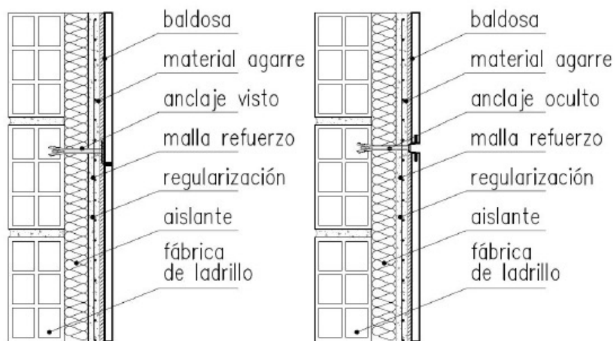
Fig.4: Detalle sistema mixto con anclaje mecánico R2m
