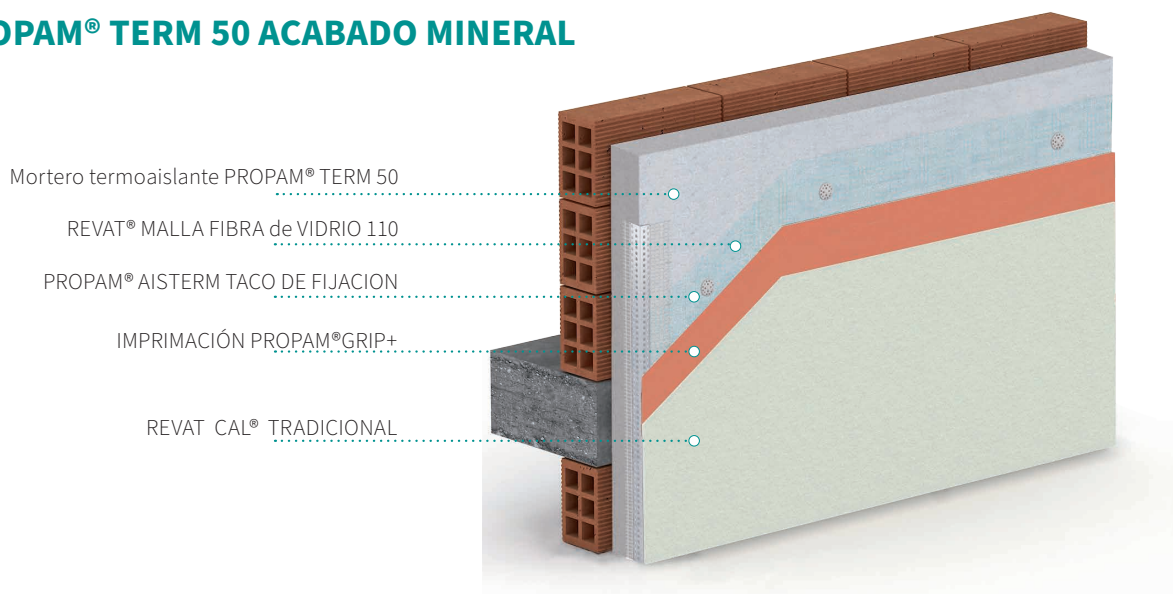
Fig.2: Sistema PROPAM® TERM 50 acabado MINERAL
