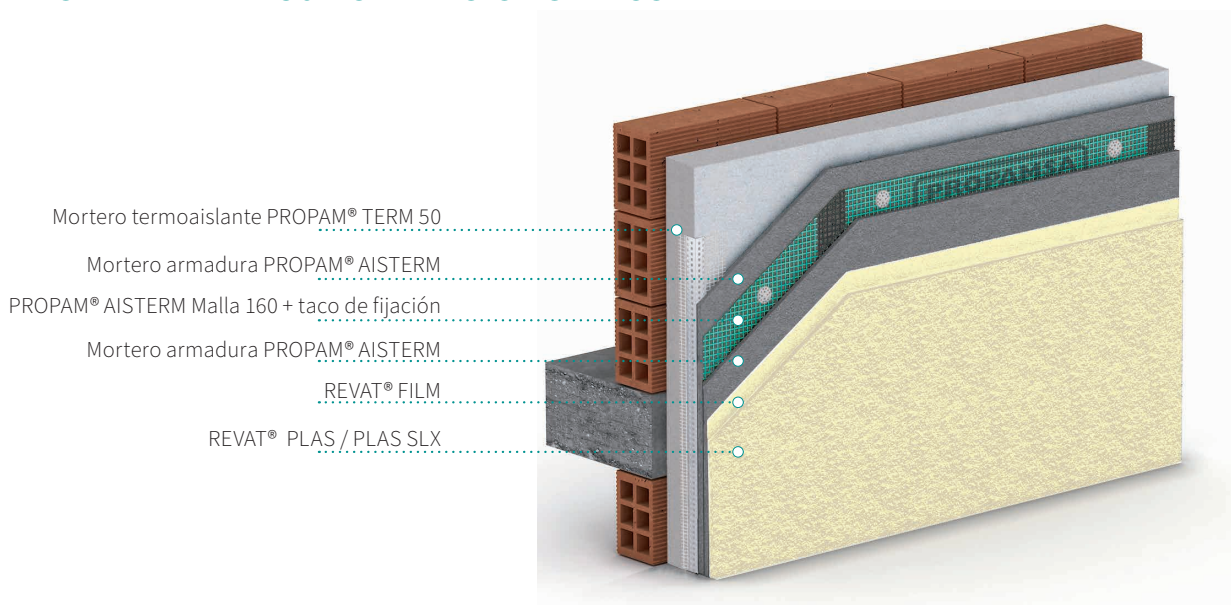
Fig.1: Sistema PROPAM® TERM 50 acabado ORGÁNICO
