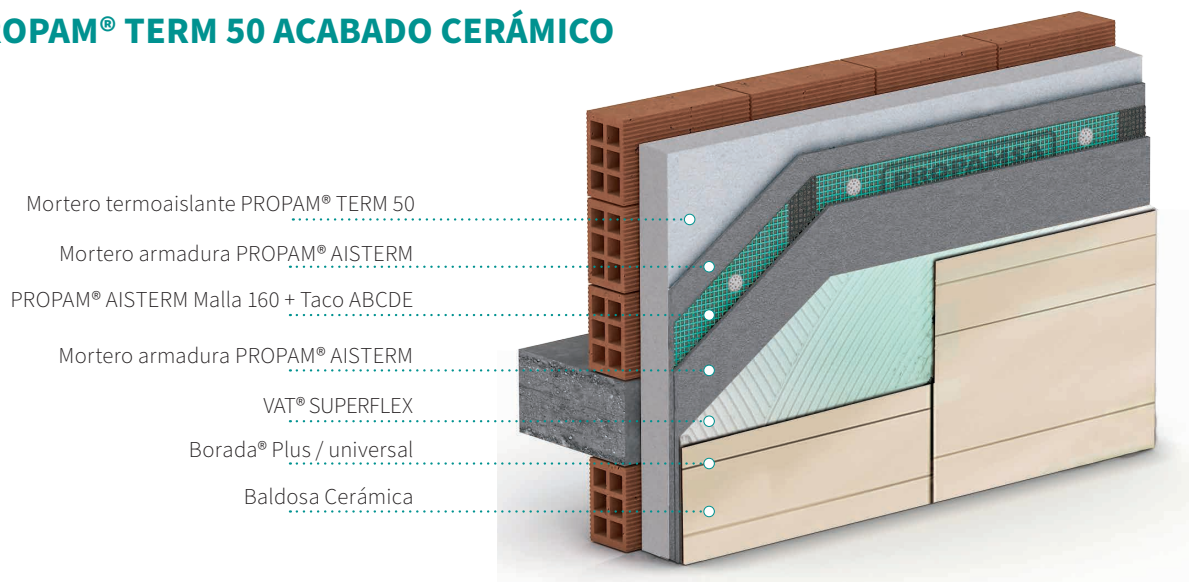
Fig.3: Sistema PROPAM® TERM 50 acabado CERÁMICO
