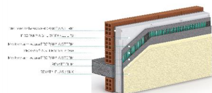
Figura 2. Configuración del sistema SATE CONFORT +
